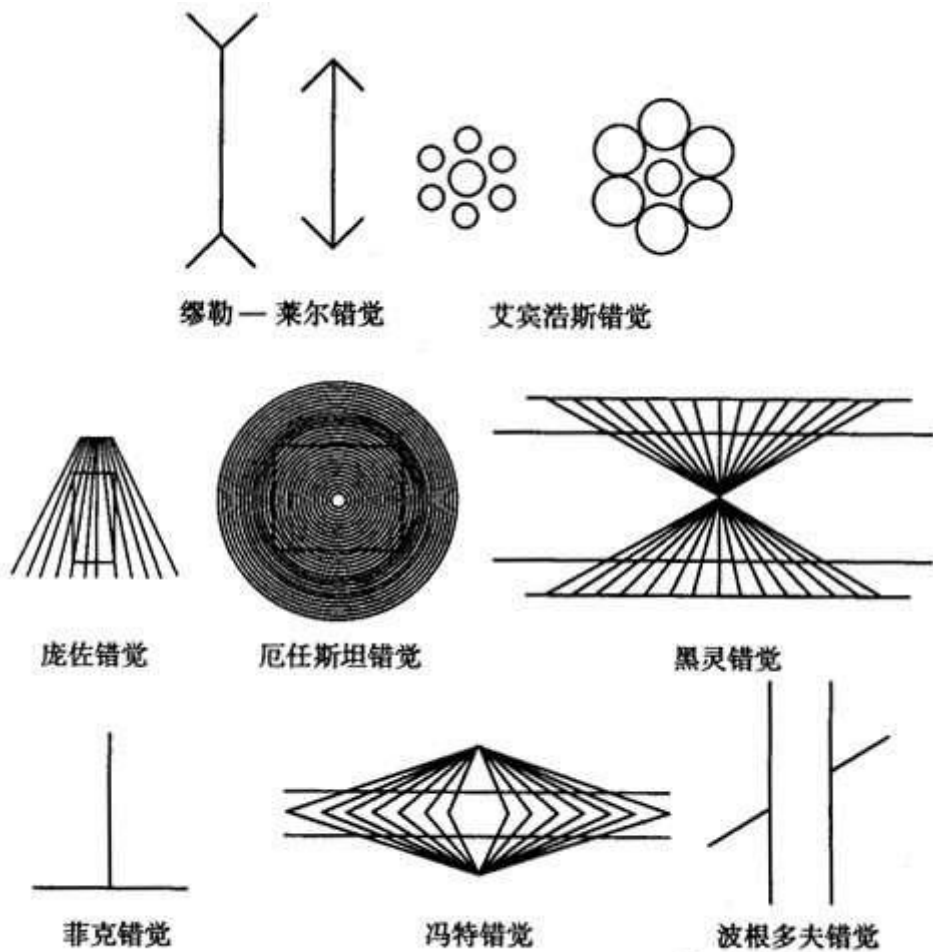
图 3-3 视错觉
